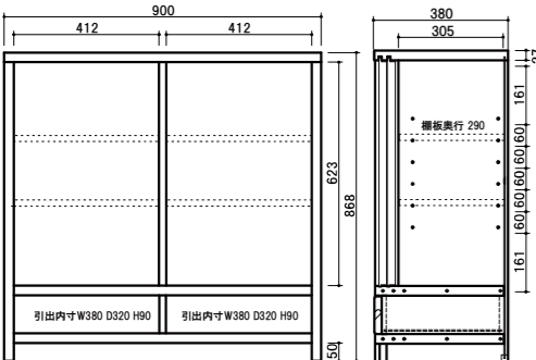
商品コード 5000 90 サイドボード WH色 商品コード 5001 120 サイドボード WH色
