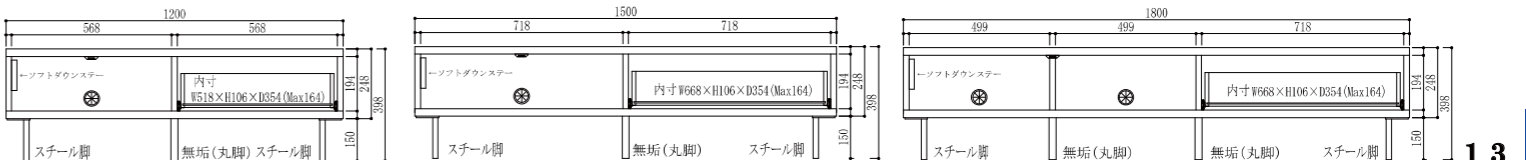
商品番号 4400 120 TV ボード WAL色 W1200 D421 H398(内脚150) 重量約34kg 才数 5.2/個口数 1 ¥76,700 [税別] 商品番号 4401 150 TV ボード WAL色 W1500 D421 H398(内脚150) 重量約46kg 才数 6.5/個口数 1 ¥86,700 [税別] 商品番号 4402 180 TV ボード WAL色 W1800 D421 H398(内脚150) 重量約58kg 才数 7.7/個口数 1 ¥100,000 [税別]
