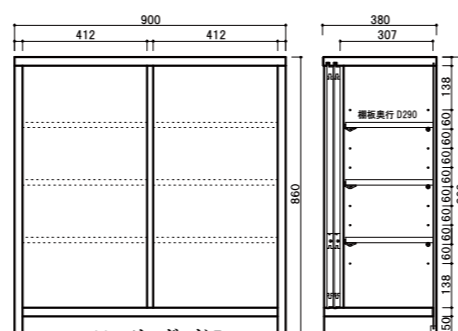
商品コード 5020 90 フリーボード L WH色 商品コード 5021 90 フリーボード H WH色
