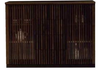
商品コード 1324 120サイドボードBR色 W1200×D435×H890 棚板4枚 裏化粧 ④⑥ 透明ガラス ¥129,000 [税別] 才数 17.5/個口数 1 約53kg
