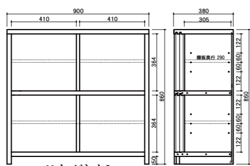
商品コード 5010 90 キャビネット L WH色 商品コード 5011 90 キャビネット H WH色
